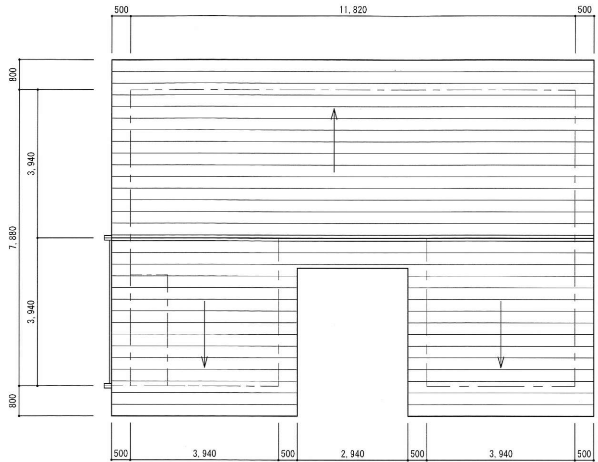
屋根伏図
