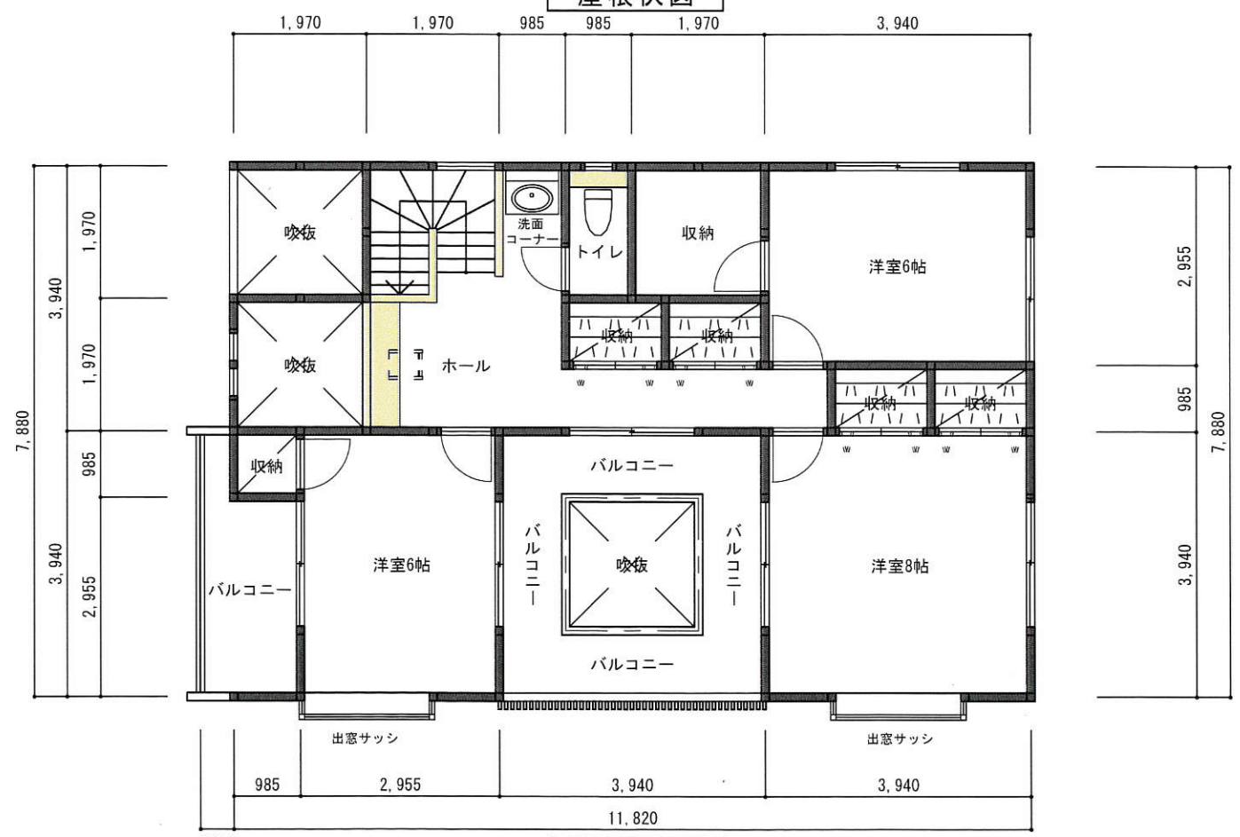
2階平面図
