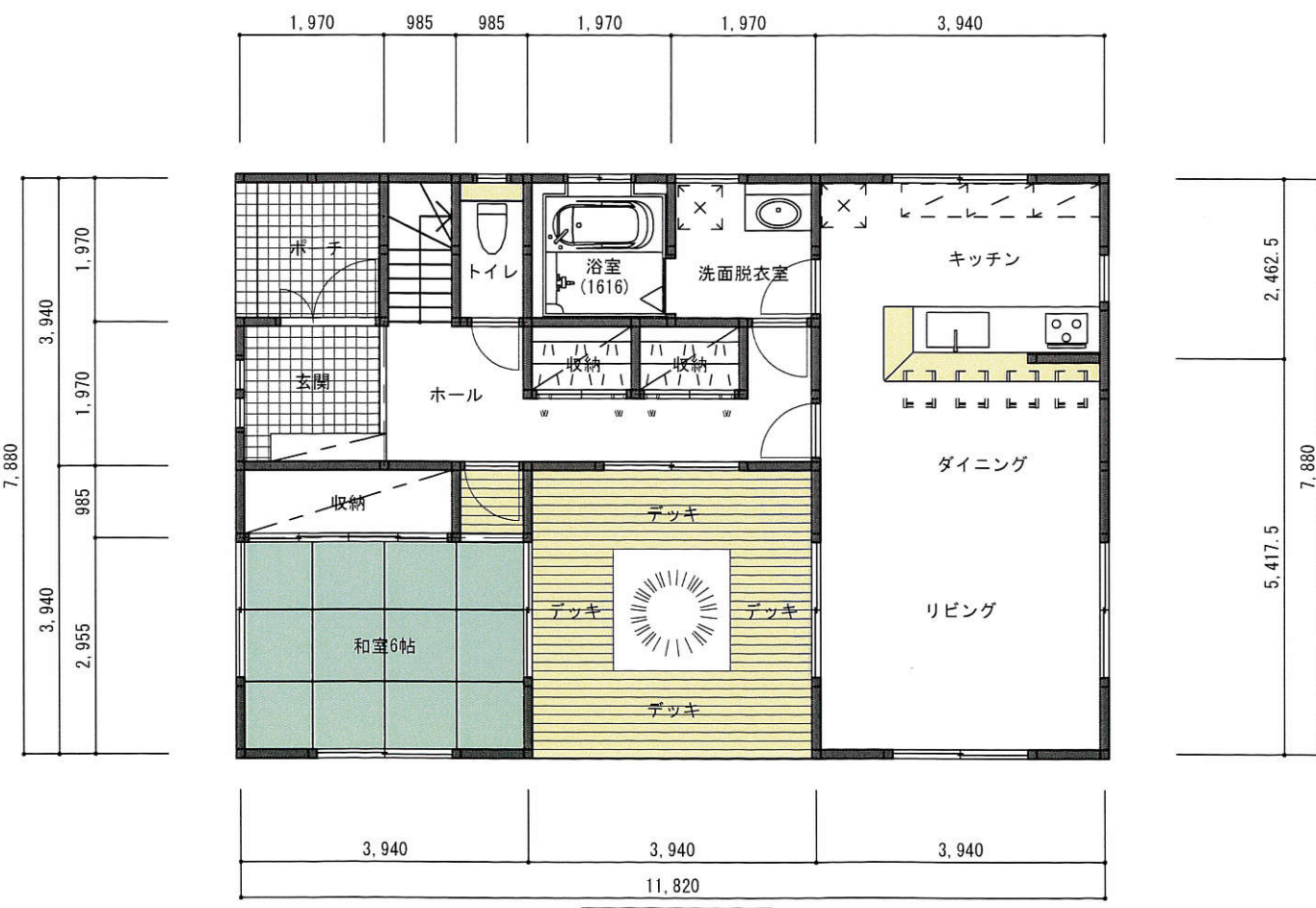
1階平面図
