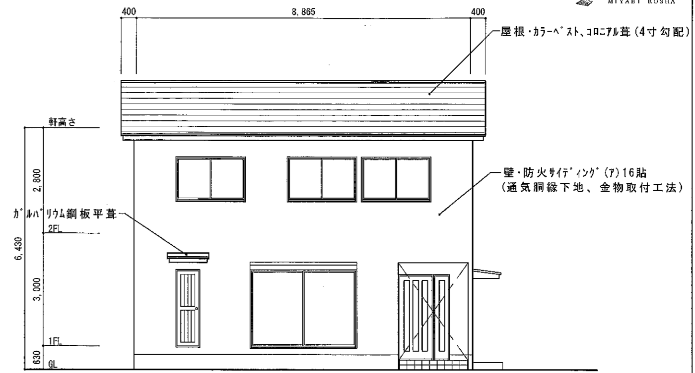
南立面図
