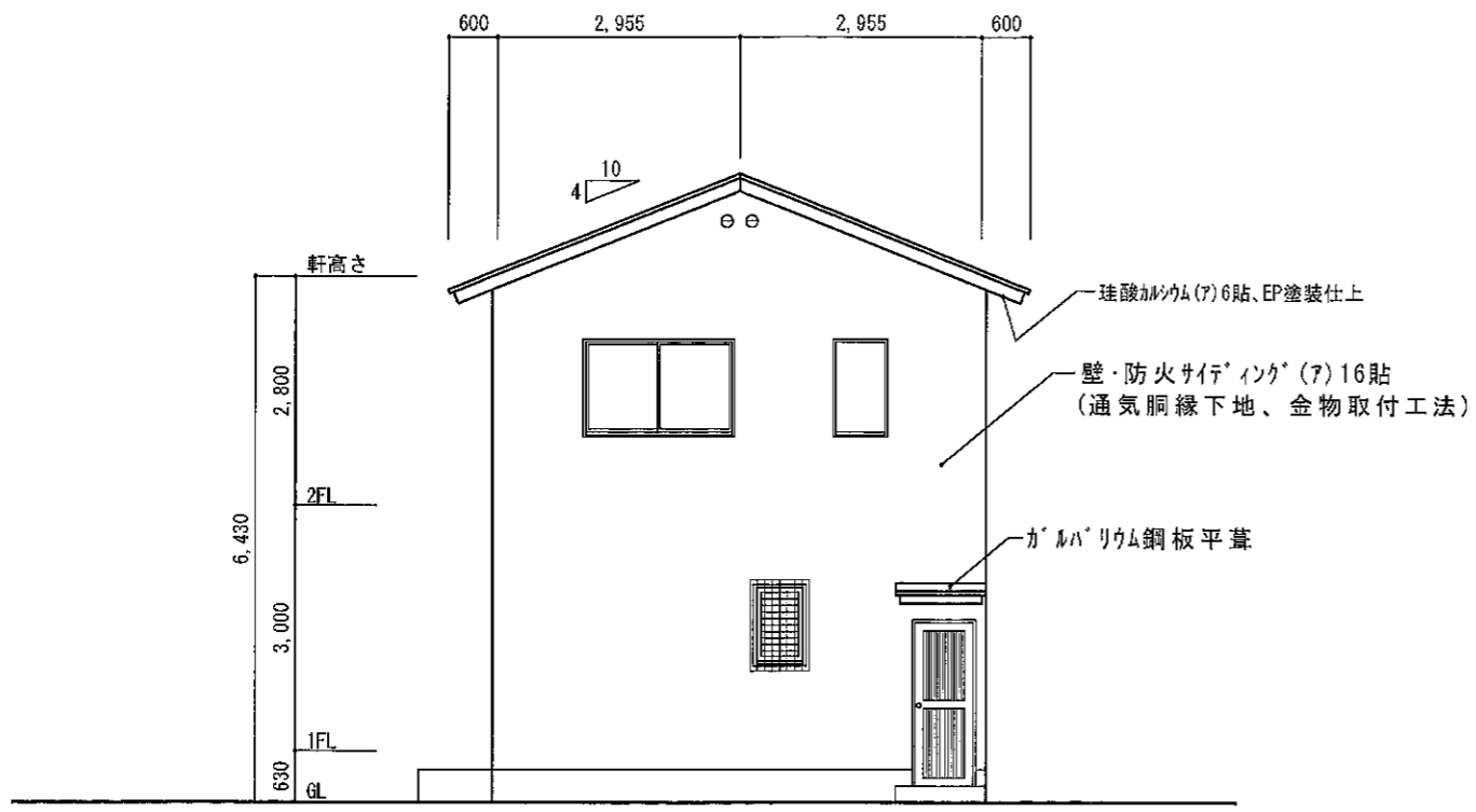
東立面図
