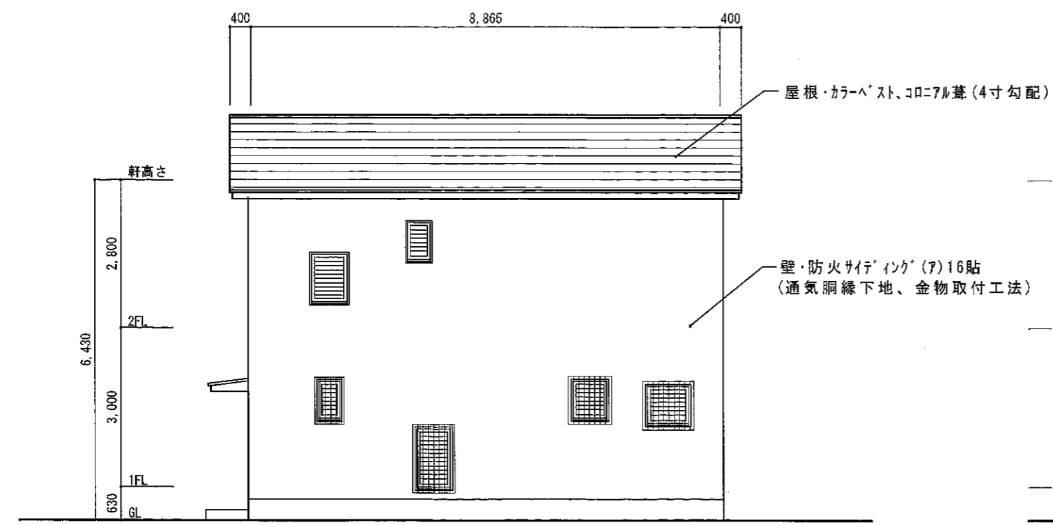
北立面図
