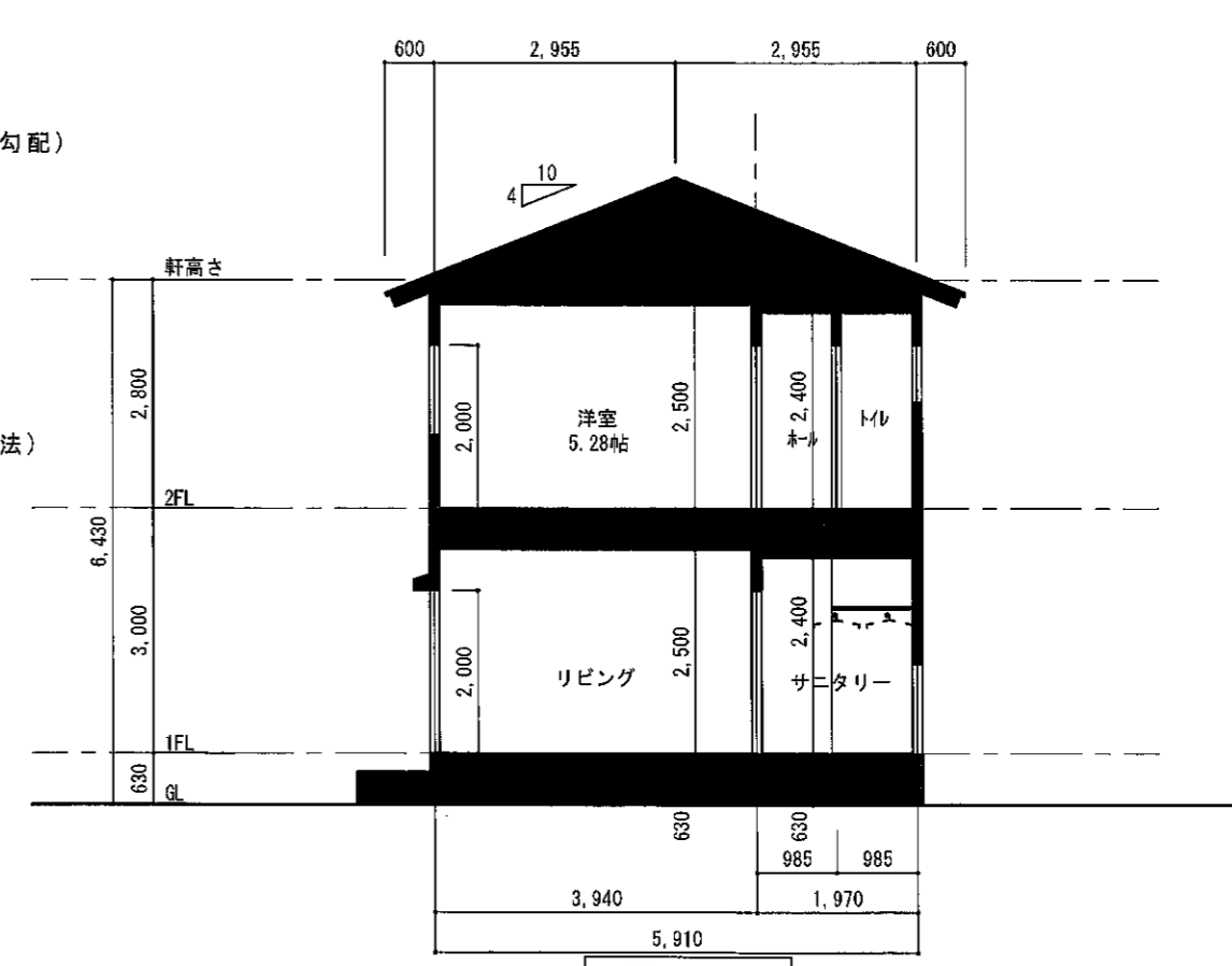
縦断面図
