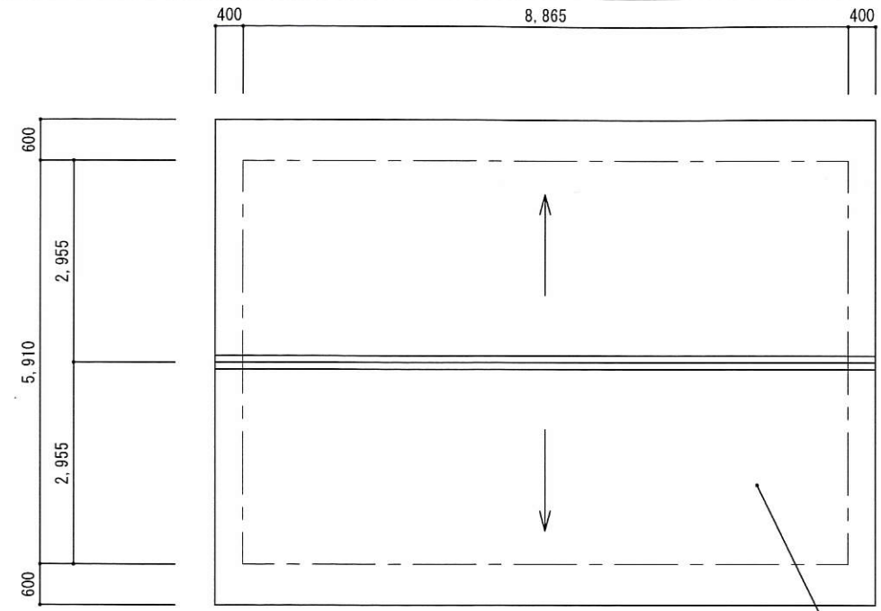
屋根伏図
